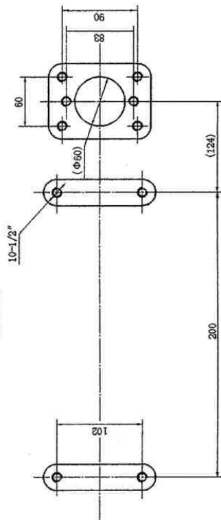
底脚尺寸
